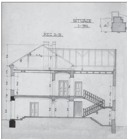
Plán na přístavbu školní budovy – řez – z roku 1907 (archiv Obce Olešanky)
