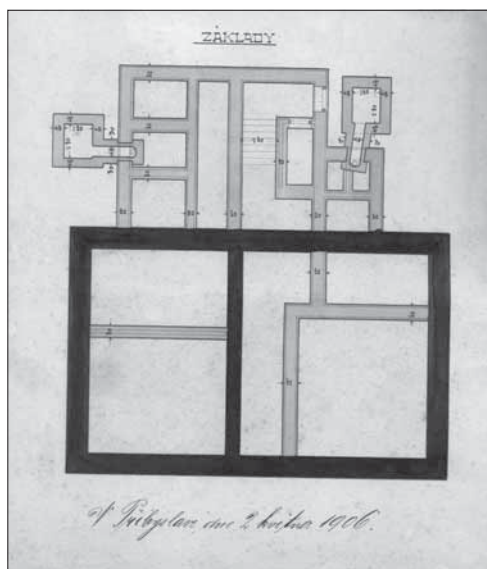
Plán na přístavbu školní budovy – základy – z roku 1907 (archiv Obce Olešanky)
