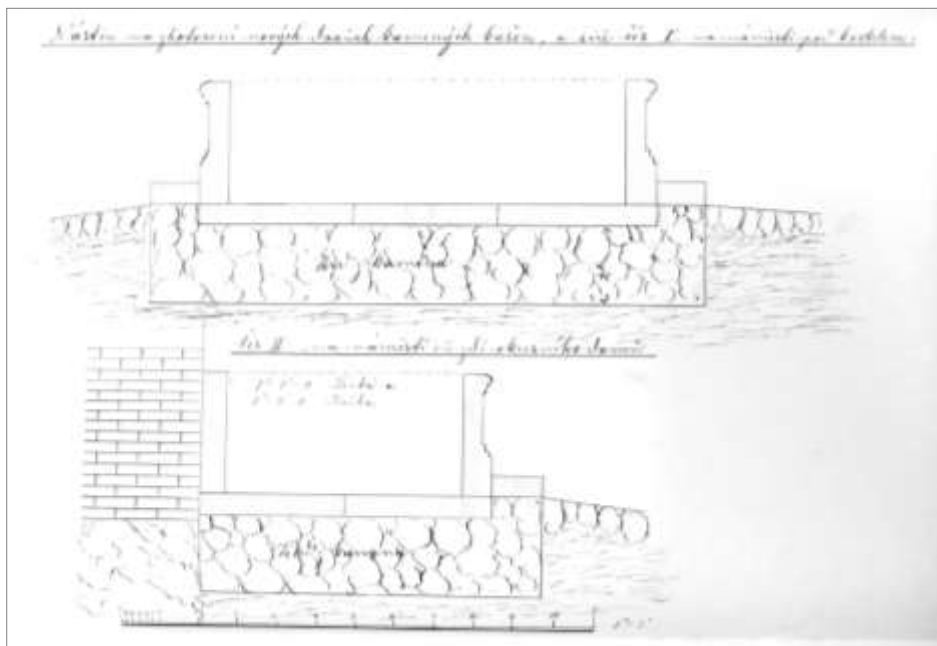
Náčrtek menší kašny k budově okresního soudu od Liberáta Kundta, 1869 (MMP)
